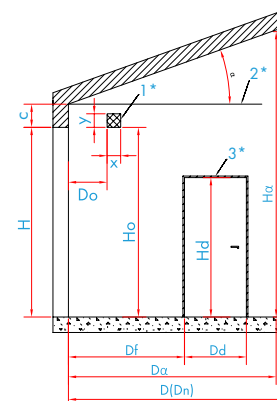
Seitenschnitt
