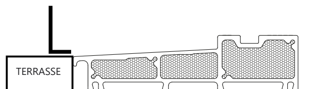
Schwelle mit Ausgleich zur Terrasse: untere Führung Typ „L“
