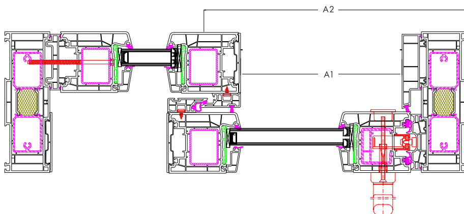
Grundriss (Ansicht von oben)
