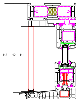
Schnitt (Ansicht von der Seite)
